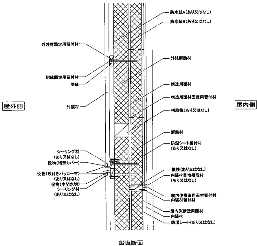
鉛直断面
