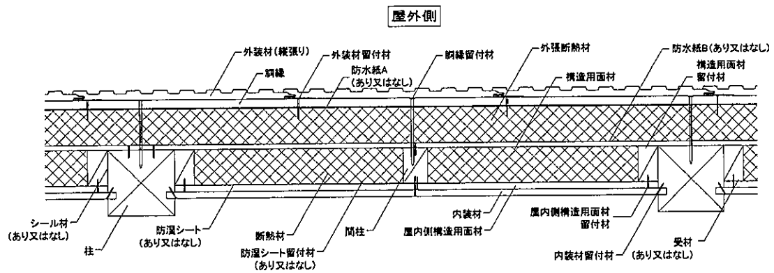
屋内側 水平断面
