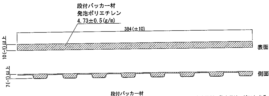
図19 構造説明図
