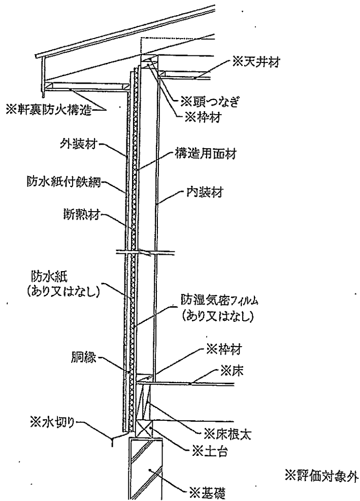
鉛直断面図
