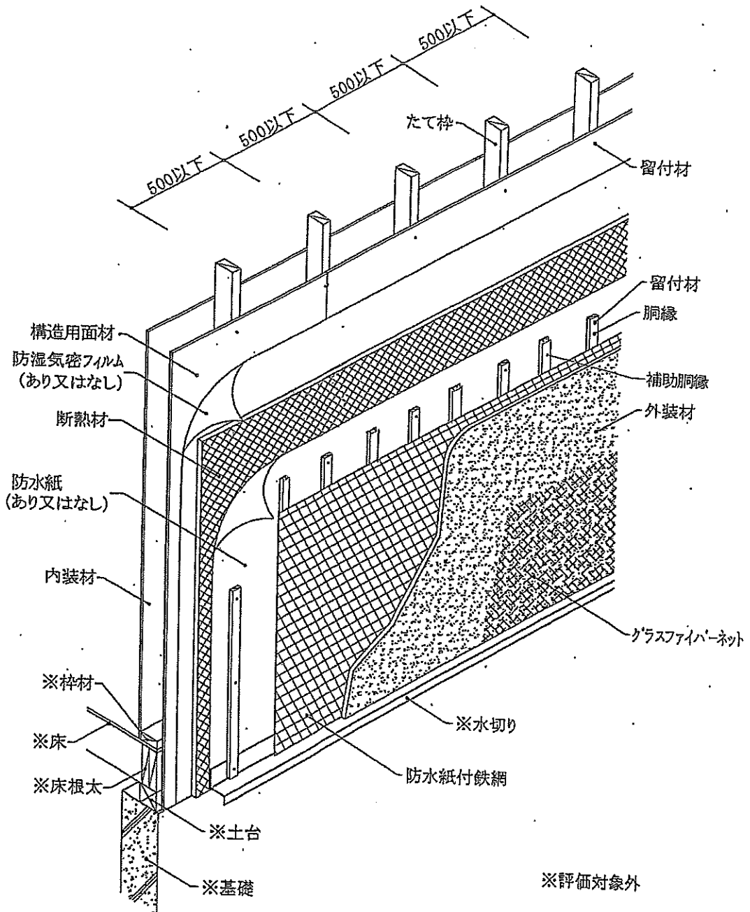
透視図
