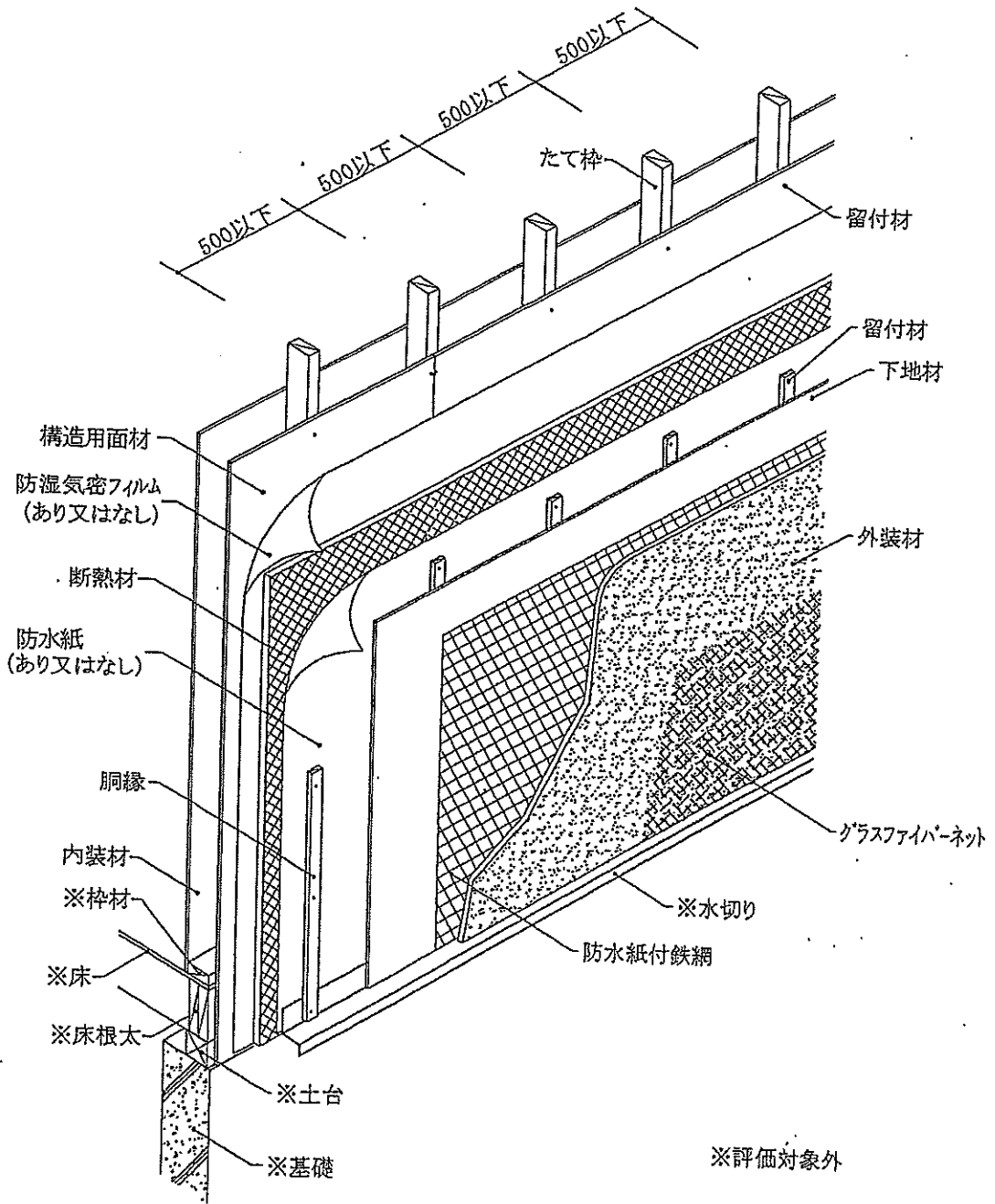
透視図
