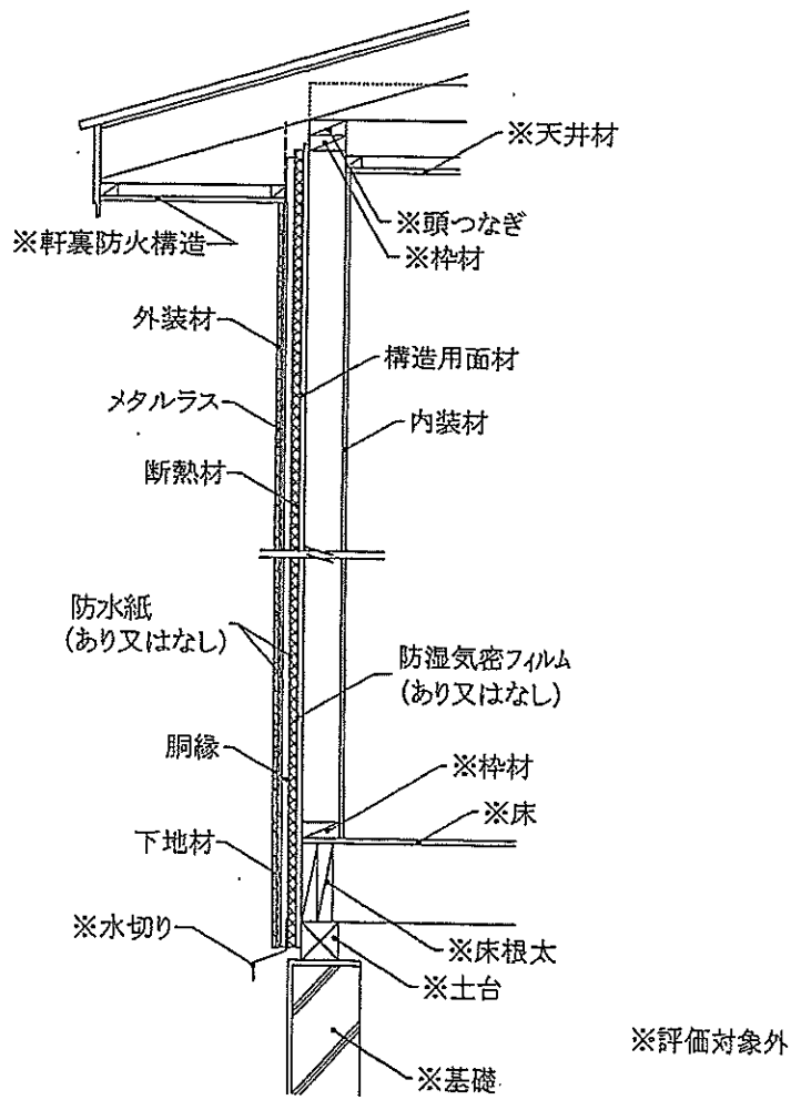
鉛直断面図
