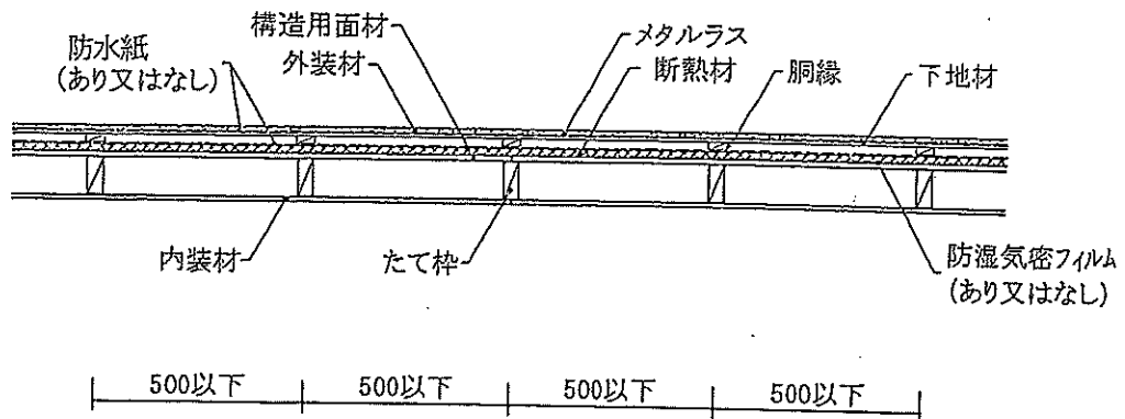
水平断面図
