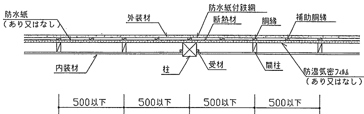
水平断面図
