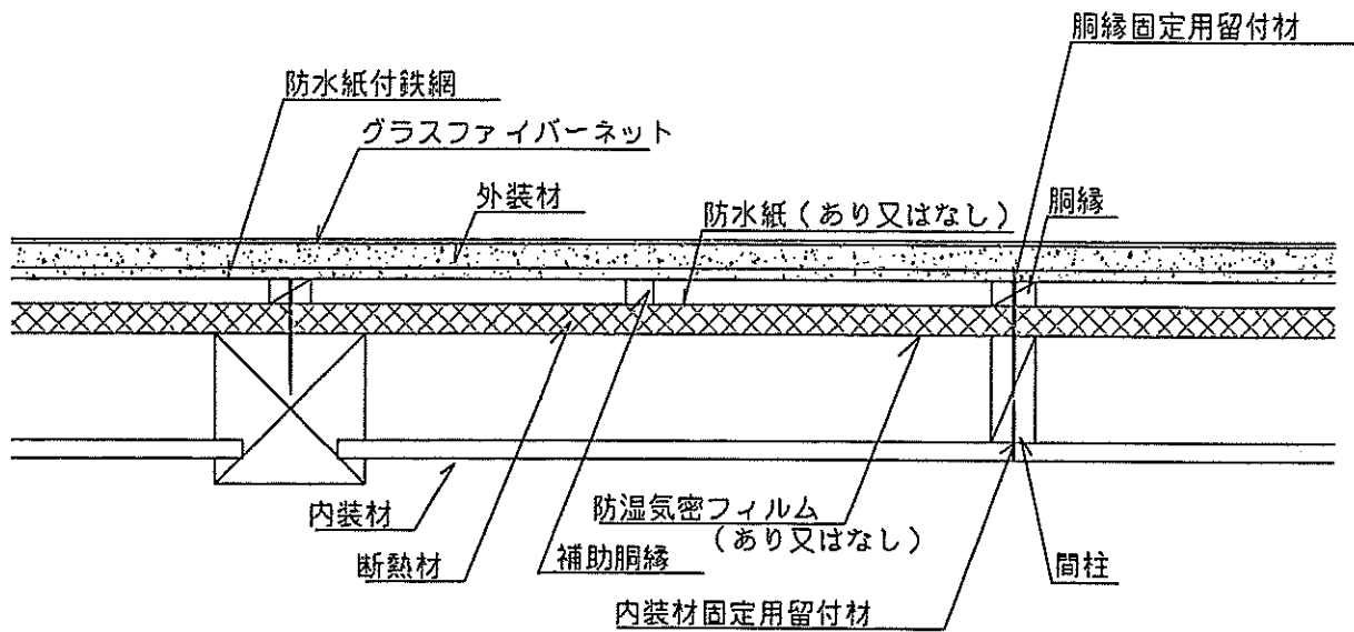
水平断面図
